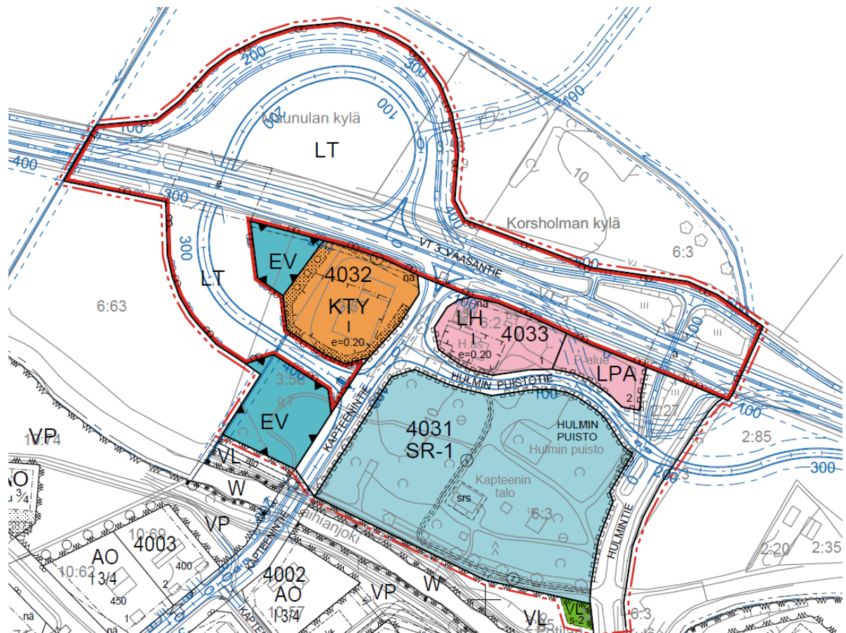
Kuva 2. Ote asemakaavaehdotuksesta tiesuunnitelmaluonnoksen (sinisellä) kanssa. Puistossa sijaitsevat rakennukset ja jäljellä olevat rakennusten jäänteet sijoittuvat asemakaavaehdotuksessa esitetyille SR-1-alueelle.
